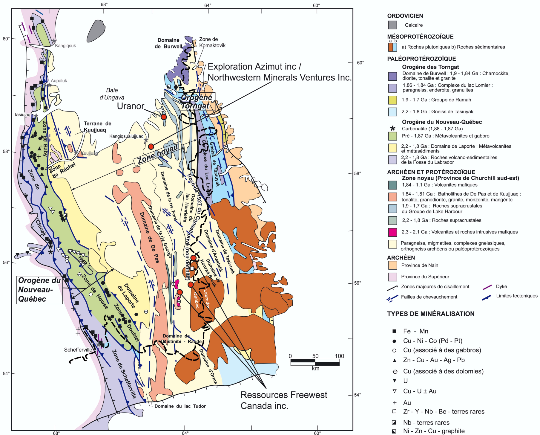
Figure 2. Sites de découvertes d'indices minéralisés (points en noirs) en U des compagnies minières actives en 2006 dans les orogènes du Nouveau-Québec et des Torngats ainsi que dans la "zone noyau". Modifiée de Wardle et al. 1990 et 2002.
