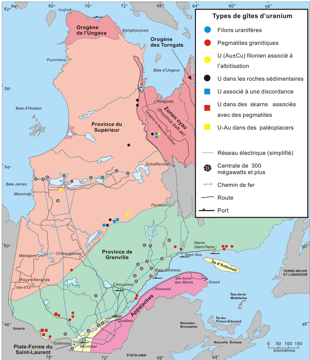
Figure 1. Subdivisions géologiques et localisation des principaux indices et gîtes d'uranium au Québec.
